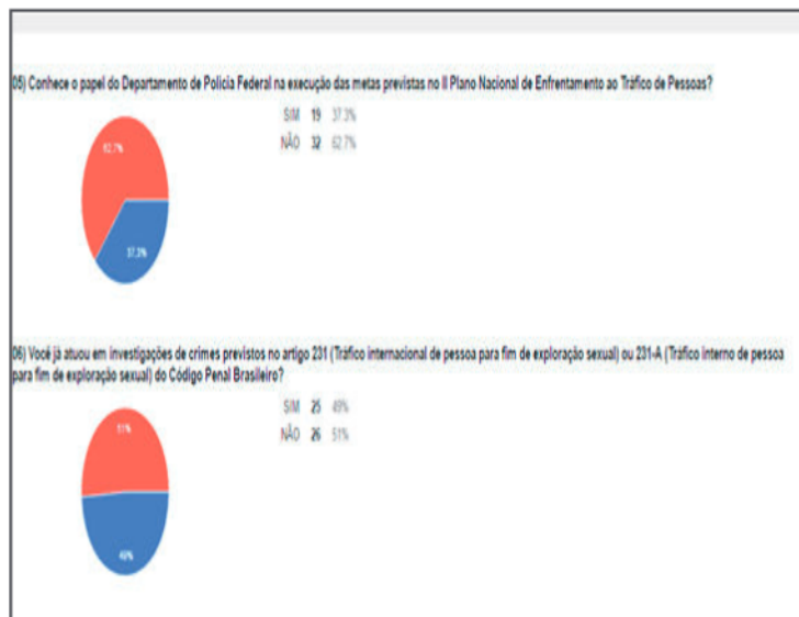
Gráfico 5 - Questionário
